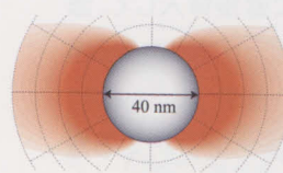
近接場光のシミュレーション (小林・石川研)
